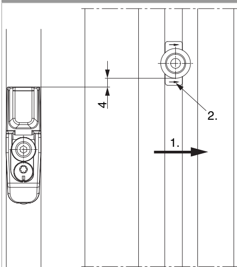
Aufsteckschließteil für i.S. Zapfen
