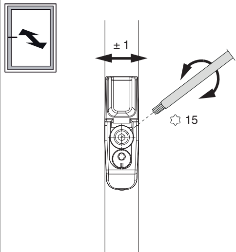
Aufsteckschließteil für i.S. Zapfen
