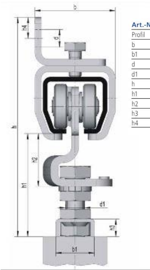
Abbildung 2. Einbauschnitt mit den Rollapparaten
