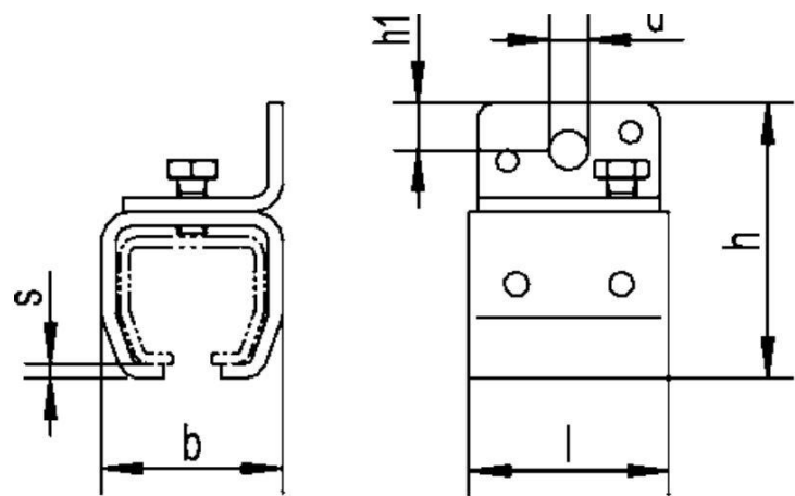
Abbildung 1 Abmessungen
