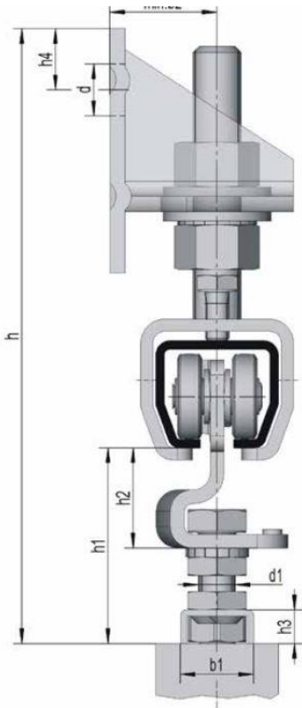
Abbildung 2. Einbauschnitt
