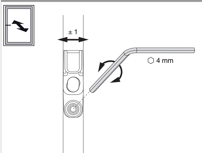
Aufsteckschließteil für VZ
