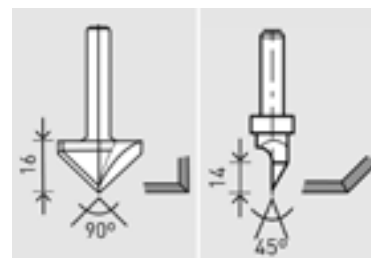
90°-Gipskartonfräser (Bestell-Nr. 491001)
