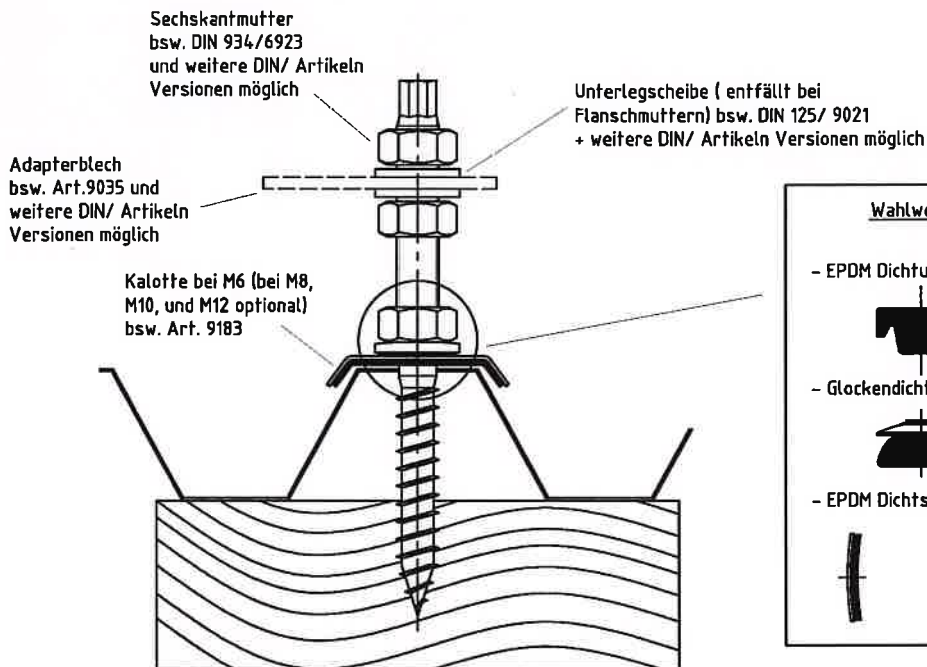
Stockschraube Standard Sechskant zwischen dem Gewinde. Durchmesser(Ø) M6, M8, M10, M12
