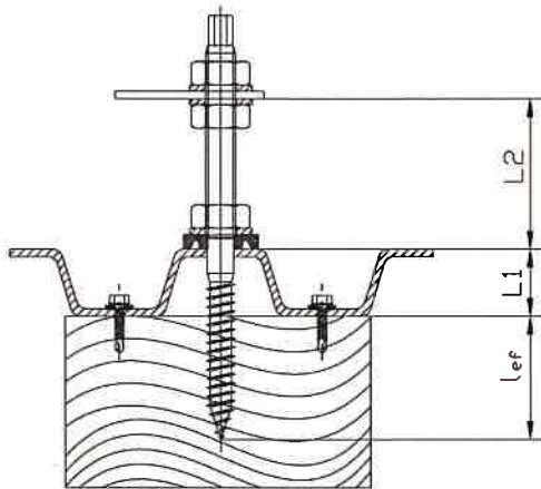
Abbildung 1: Befestigung der Profiltafeln bei Verwendung der "S + P" Stockschrauben
