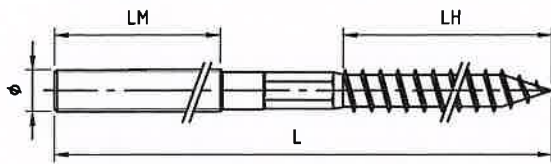
Stockschraube Standard Sechskant zwischen dem Gewinde. Durchmesser(Ø) M6, M8, M10, M12
