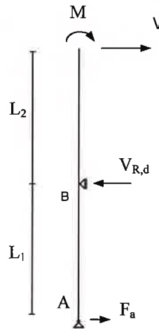
Abbildung 3: Statisches System der "S + P" Stockschräuben
