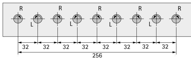
Bohrbild
