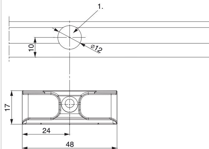
Bohrbild
