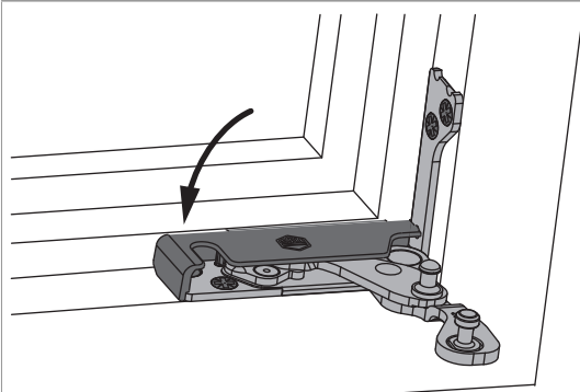
3. Abdeckkappe in Grundplatte einklipsen. • Falzluft unten waagrecht mindestens 12 mm!
