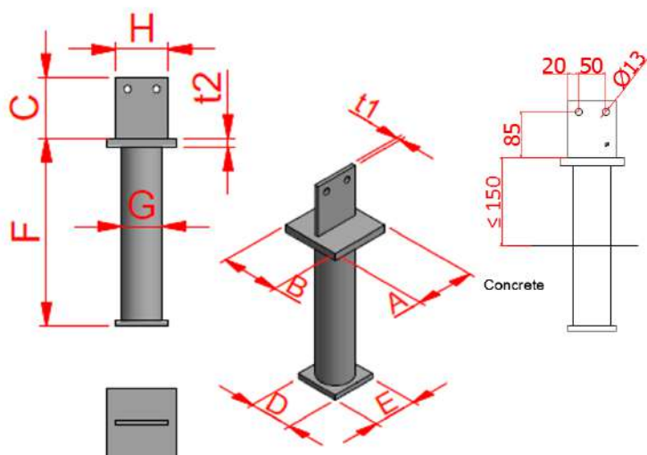
PIS70
