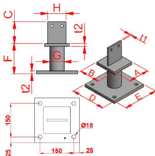
PISBMAXI
