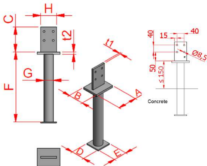
PIS70
