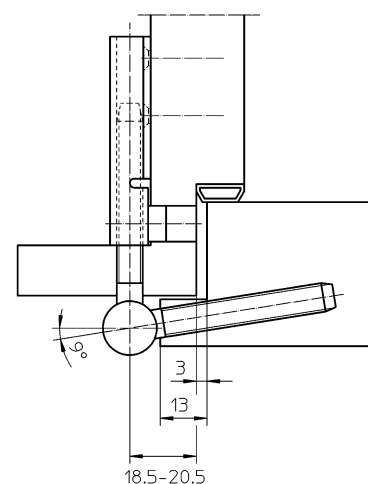
Querschnitt
