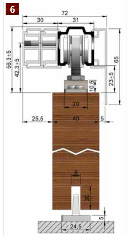
HELM 73 – Wandmontage, mit seitlich gebohrter Laufschiene, doppeltem Abstandsprofil und einsei- tiger Verblendung Beschlagzusammenstellung siehe Seite 27
