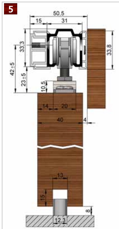
HELM 73 – Wandmontage, mit seitlich gebohrter Laufschiene, Abstandsprofil und einseitiger Verblen- dung (Holzverblendung bauseits) Beschlagzusammenstellung siehe Seite 27
