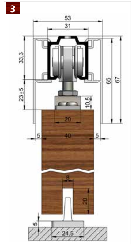
HELM 73 – Deckenmontage, mit beidseitiger Verblendung Beschlagzusammenstellung siehe Seite 26
