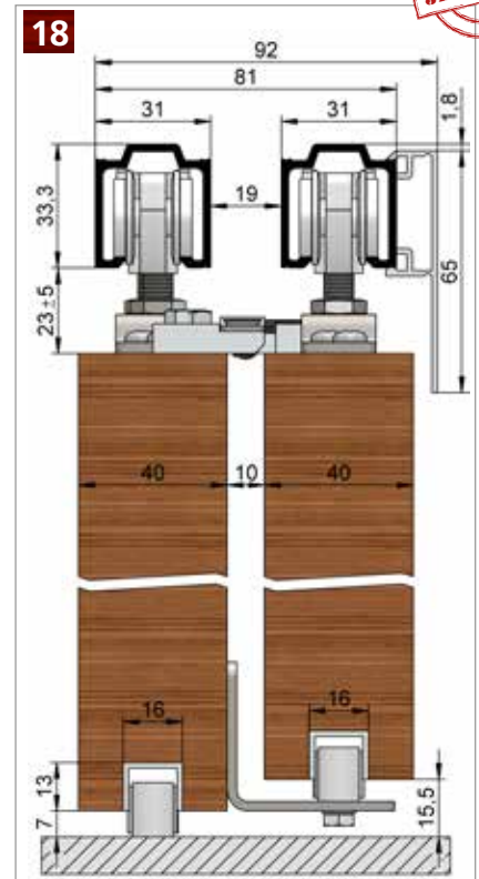
HELM 73 – Deckenmontage , Teleskopbeschlag mit unterer HELM 240 Führungsschiene, HELM SmartGuide H 216 S und HELM SmartGuide H 216 S mit Befestigungswinkel Beschlagzusammenstellung siehe Seite 29
