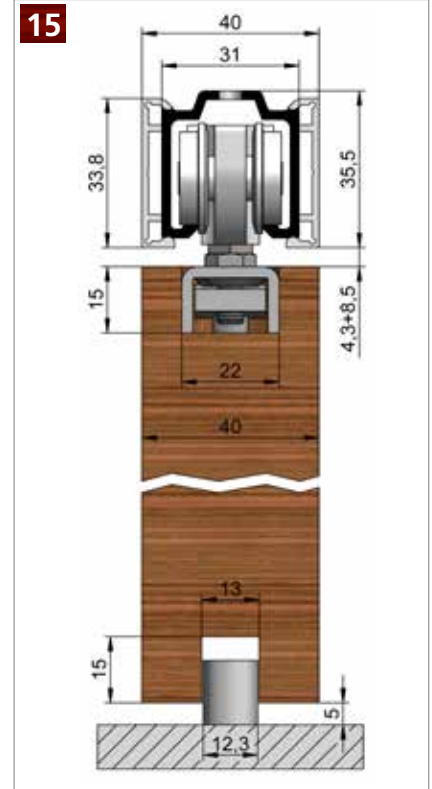
HELM 73 ME- V – Deckenmontage , mit minimaler Einbauhöhe und beidseitiger ME Verblendung Beschlagzusammenstellung siehe Seite 29
