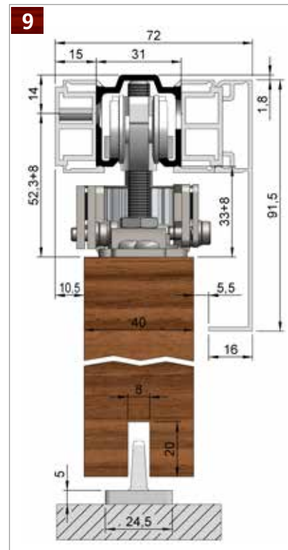
HELM 73 – Wandmontage , synchron mit Blende zum Aufklipsen, seitlich gebohrter Laufschiene, Abstandsprofil beidseitig und einseitiger Verblendung Beschlagzusammenstellung siehe Seite 28
