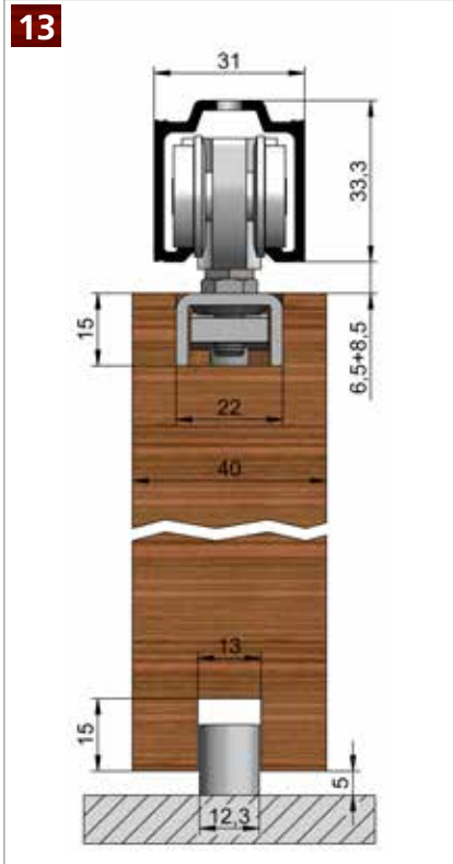
HELM 73 ME- V – Deckenmontage , mit minimaler Einbauhöhe Beschlagzusammenstellung siehe Seite 29
