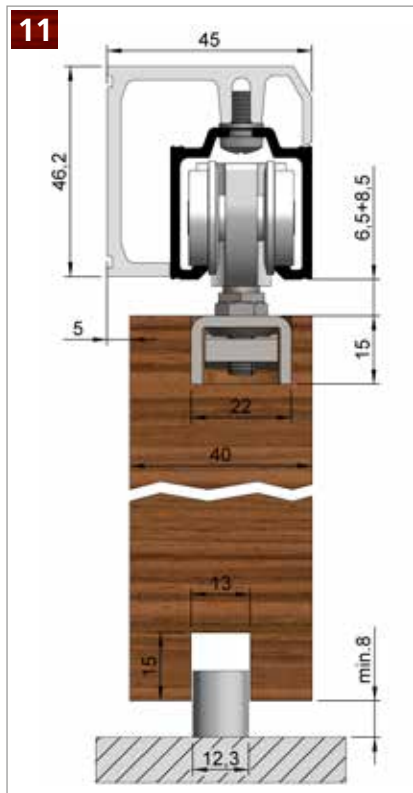
HELM 73 ME-V – Wandmontage , minimale Einbauhöhe mit Montageschiene Beschlagzusammenstellung siehe Seite 28
