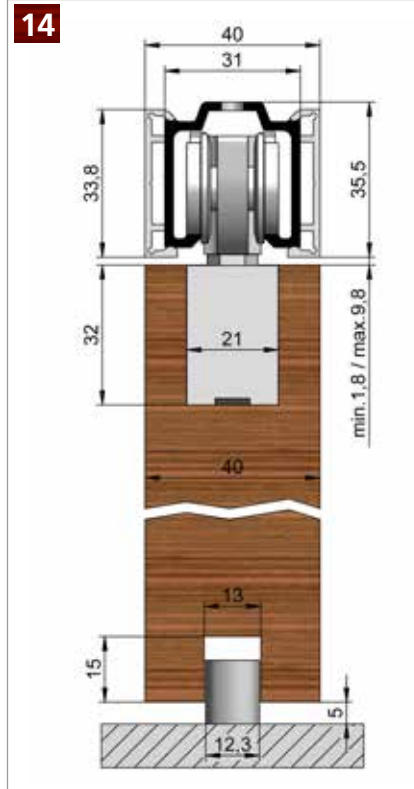
HELM 73 ME- A – Deckenmontage , mit minimaler Einbauhöhe und beidseitiger ME Verblendung Beschlagzusammenstellung siehe Seite 29
