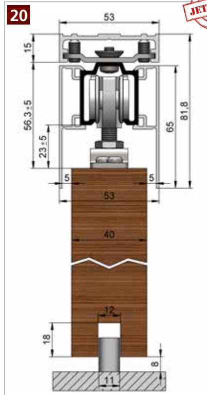
HELM 73 WT – Wandtaschenmontage mit Befestigungsschiene Beschlagzusammenstellung siehe Seite 30
