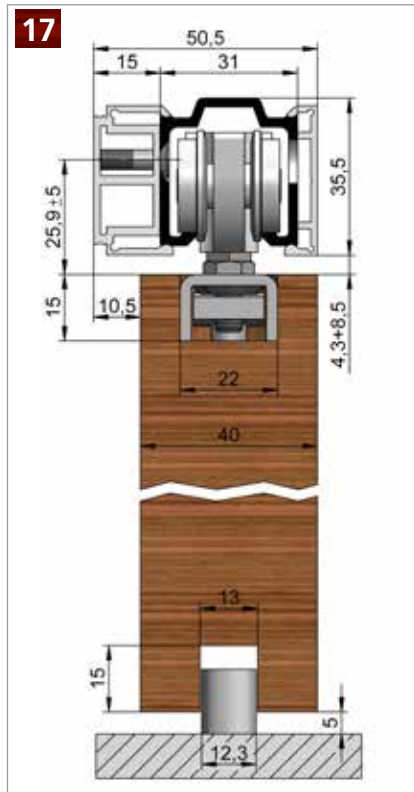
HELM 73 ME- V – Wandmontage , mit minimaler Einbauhöhe, seitlich gebohrte Laufschiene, Abstandsprofil und einseitiger ME Verblendung Beschlagzusammenstellung siehe Seite 29
