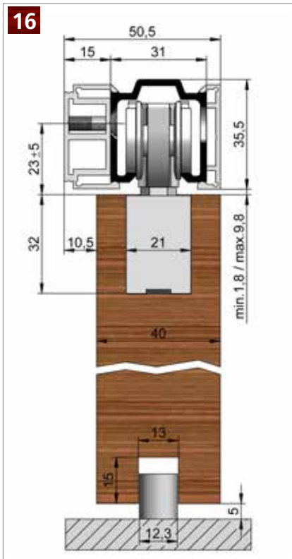
HELM 73 ME- A – Wandmontage , mit minimaler Einbauhöhe, seitlich gebohrte Laufschiene, Abstandsprofil und einseitiger ME Verblendung Beschlagzusammenstellung siehe Seite 29
