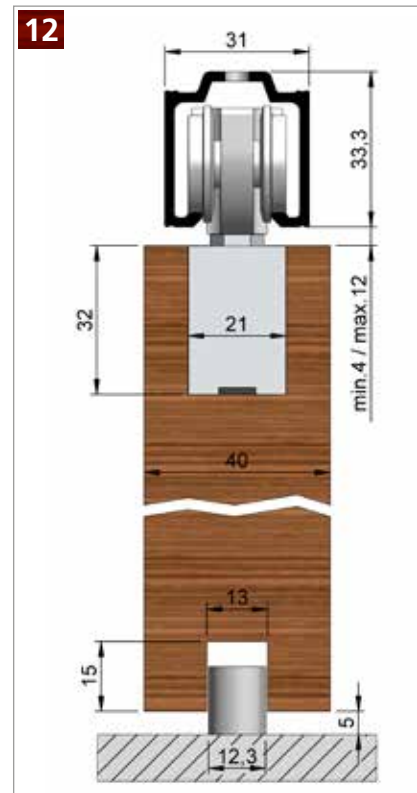
HELM 73 ME-A – Deckenmontage , mit minimaler Einbauhöhe Beschlagzusammenstellung siehe Seite 29
