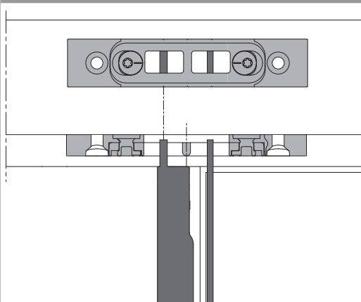
2 flg. Fenster mit 2 Stangenausschlüssen
