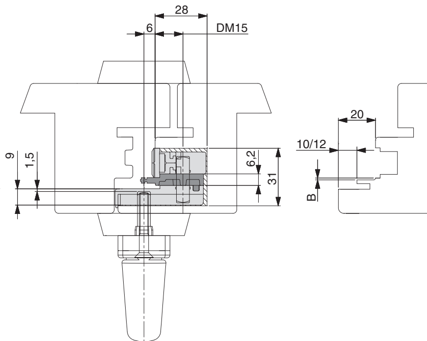
Stückliste zu Profil 12L-20Ü-9V mit kleiner Überschlagsdichtung
